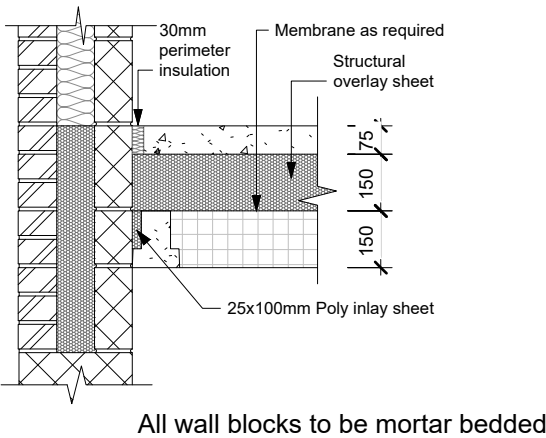
JF112 - Beam-Tight Edge Detail
